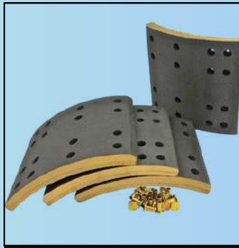
BREAK LINING VL 88 (YSM 1486)
